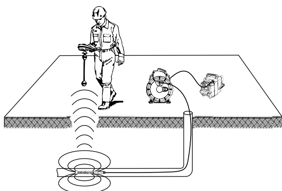
Рис. 19 - Определение местонахождения зонда катушки
