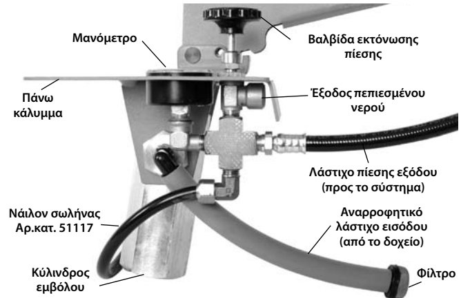
Εικόνα 2 – Εξαρτήματα αντλίας
