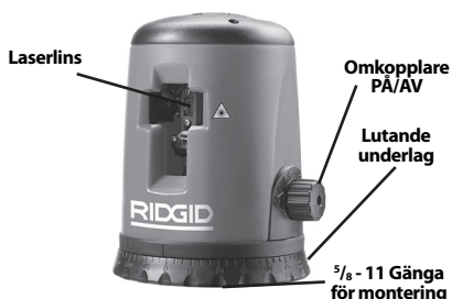
Figur 2 - Laserns delar
