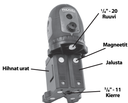
Kuva 6 - Jalusta
