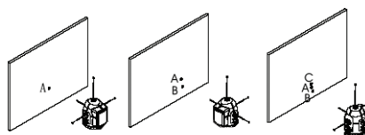
Kuva 9 - 3 vaakasäteen itsetarkastus
