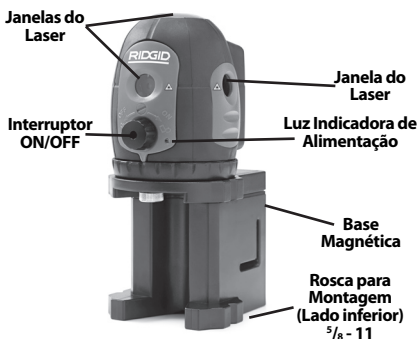
Figura 2 - Partes do Laser
