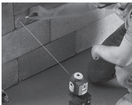
Figuur 7 – Gebruik de montageband om de Laser op zijn plaats te houden
