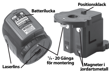
Figur 3 - Punktlaserns delar
