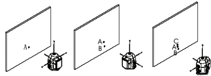
Slika 9 - Samostalna provjera 3 vodoravna snopa
