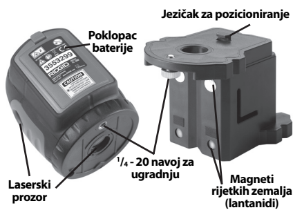
Slika 3 - Dijelovi laserskog nivelira
