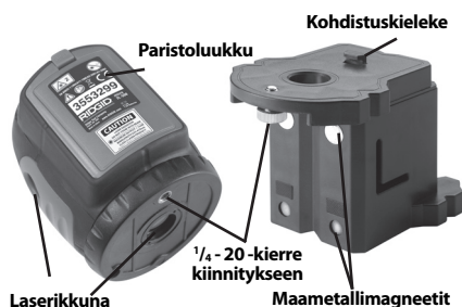
Kuva 3 - Laserin osat
