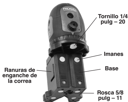
Figura 6 - Base
