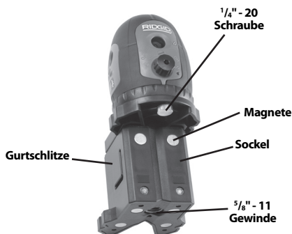
Abbildung 6 - Sockel
