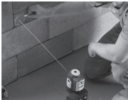
Kuva 7 - Kiinnityshihnan käyttö laserin pitämiseksi paikallaan
