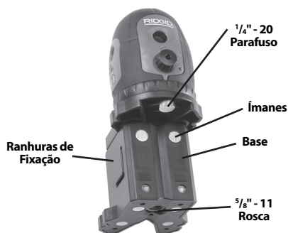
Figura 6 - Base
